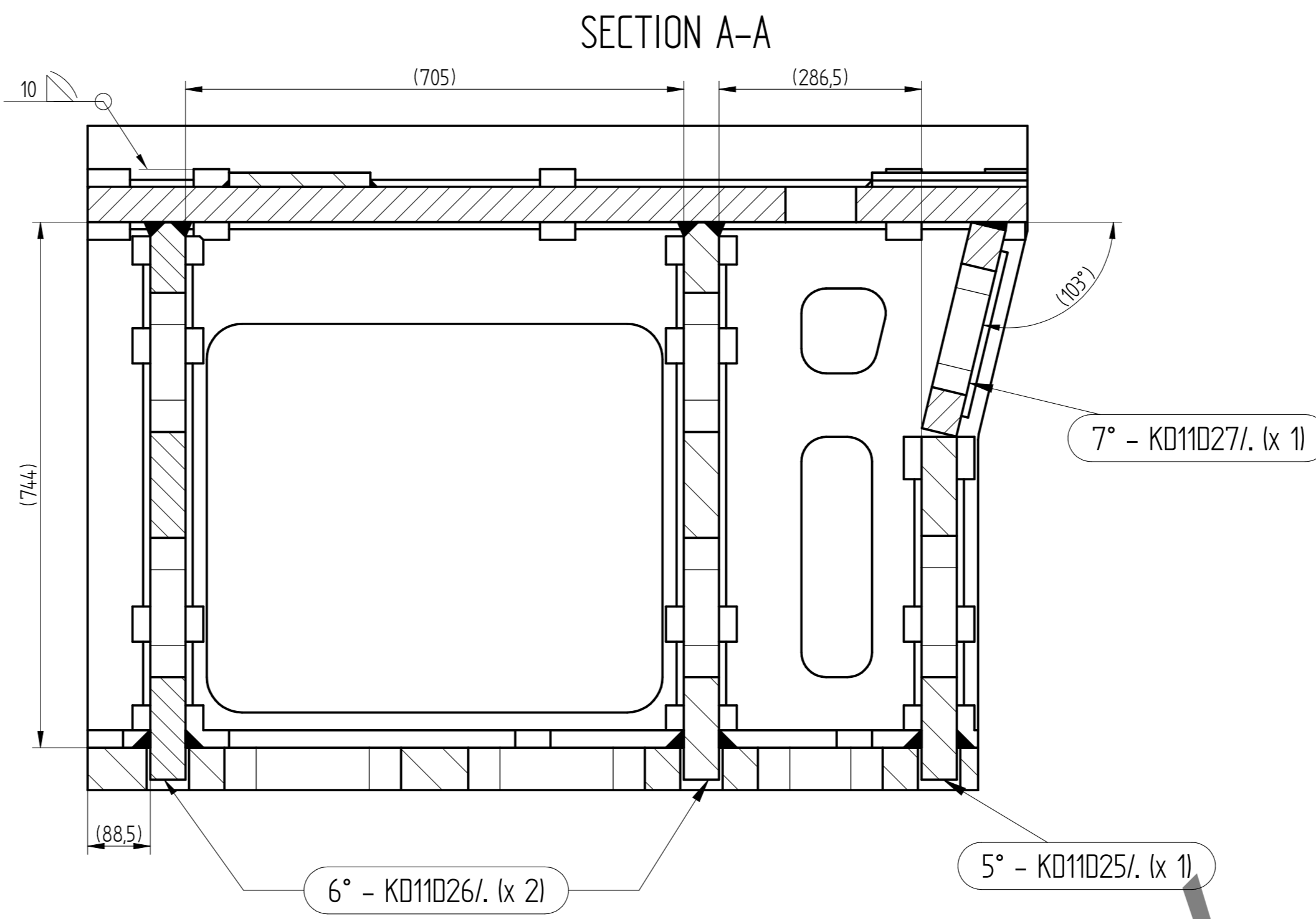
Assemblage des pièces de n° 1 à 7
